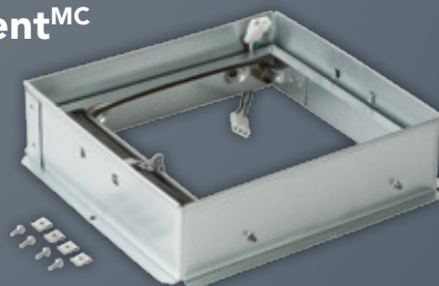
Modèle RDM1 Registre coupe-feu
